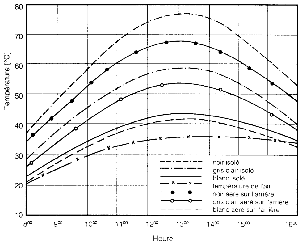
Courbe de température des plaques en PVC rigide en fonction de la couleur et de l'aération épaisseur des plaques 3-4 mm, influence de l'ensoleillement, température max. de l'air 36 °C
